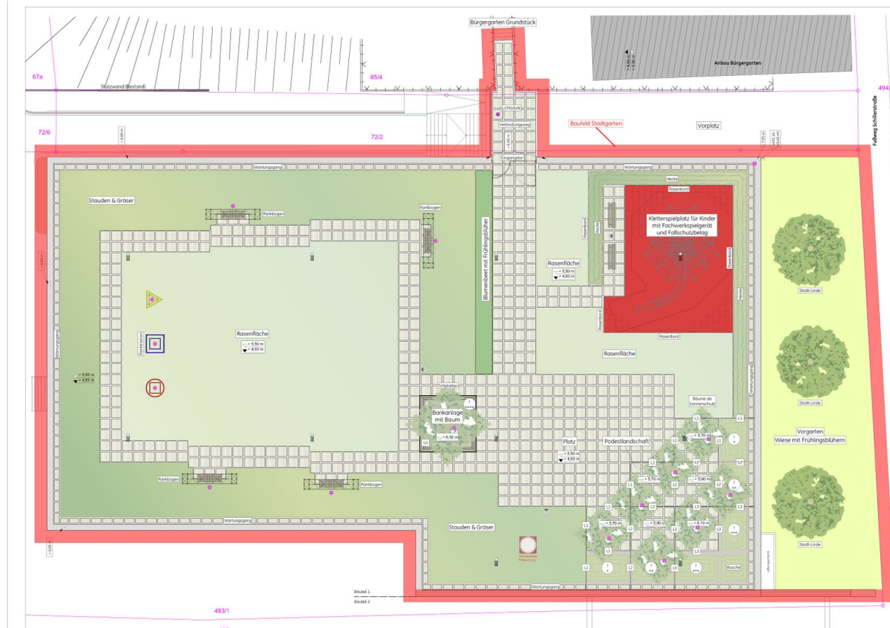
Lageplan, Entwurfsplanung Quelle: Planungsbüro Dietrich GbR
